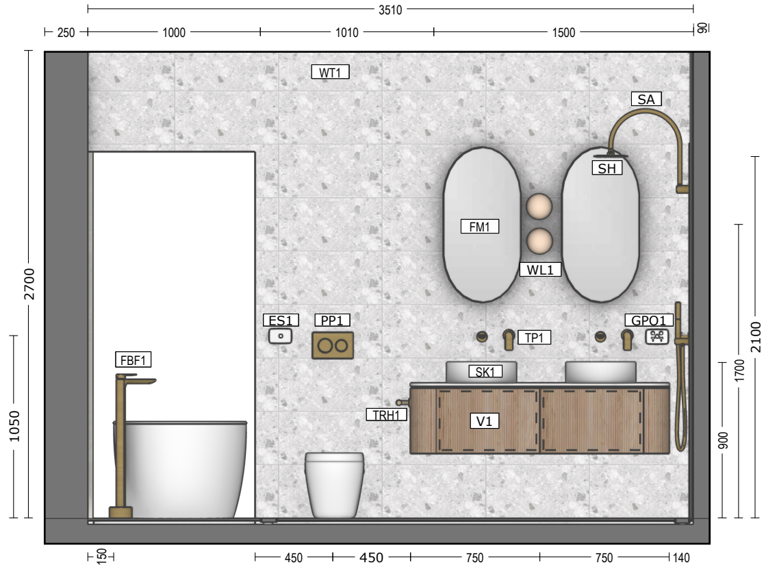
4 BATHROOM ELEVATION 04 A104 Scale: 1 : 30
