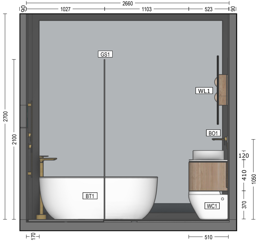
3 BATHROOM ELEVATION 03 A104 Scale: 1 : 30
