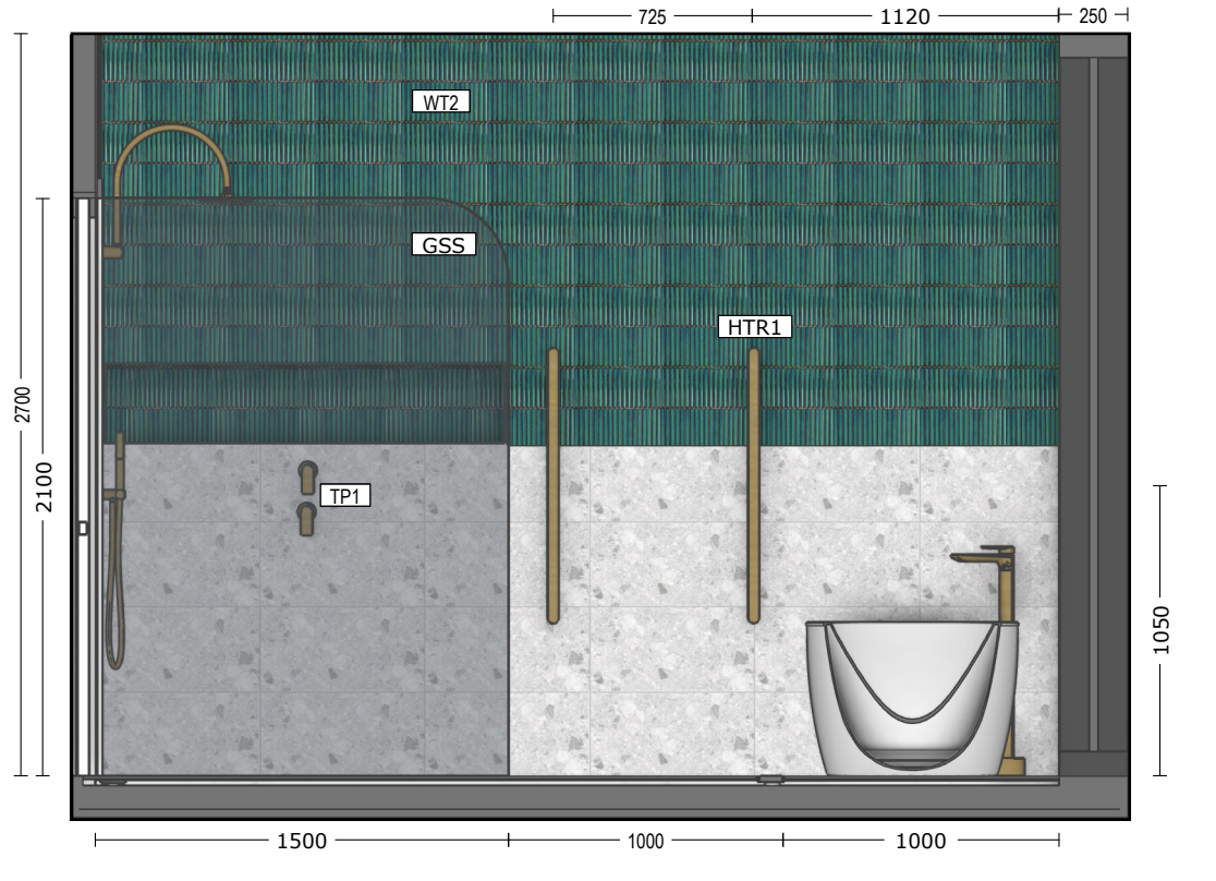
4 BATHROOM ELEVATION 04 A104 Scale: 1 : 30
